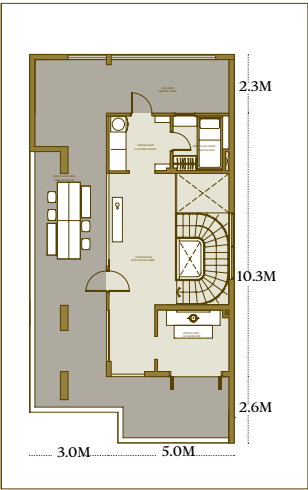
TẦNG 4 LEVEL 4
