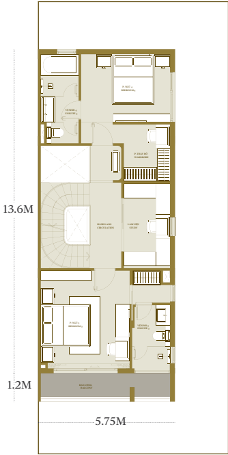
TẦNG 3 LEVEL 3
