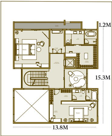
TẦNG 2 LEVEL 2
