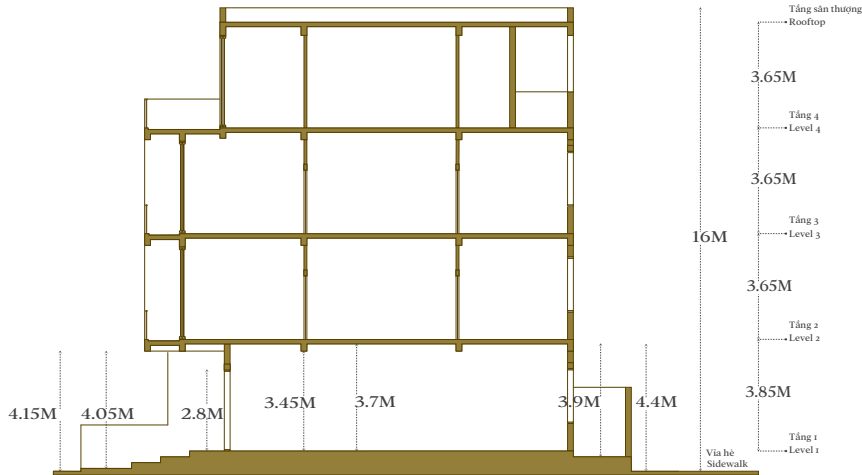
MẶT CẮT SECTION
