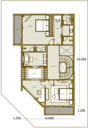
TẦNG 1 LEVEL 1
