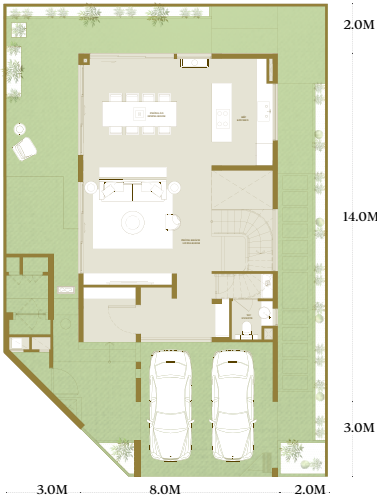
TẦNG 1 LEVEL 1
