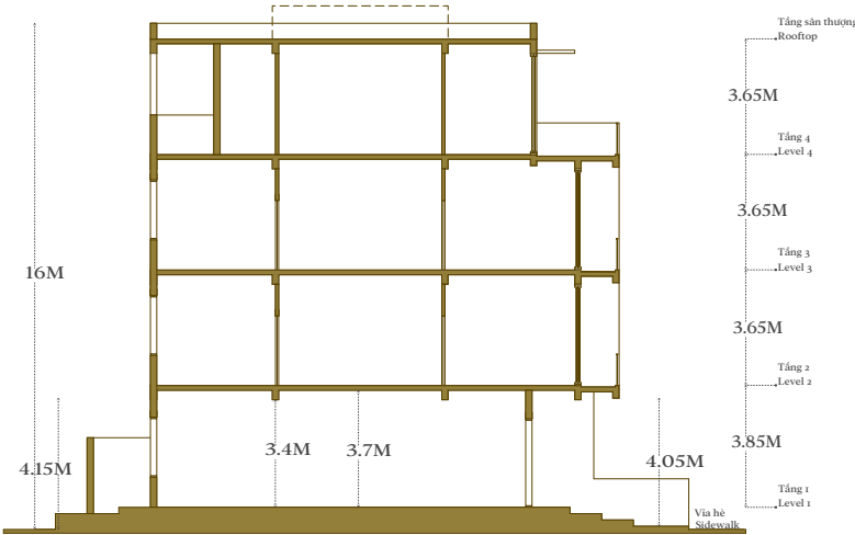
MẶT CẮT SECTION
