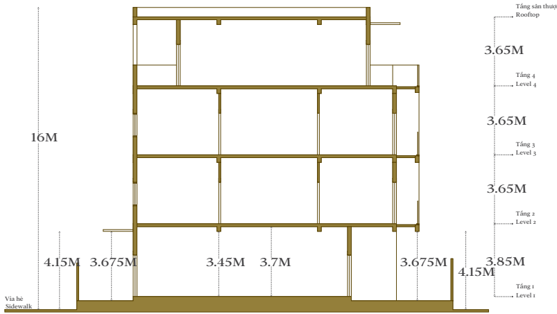
MẶT CẮT SECTION
