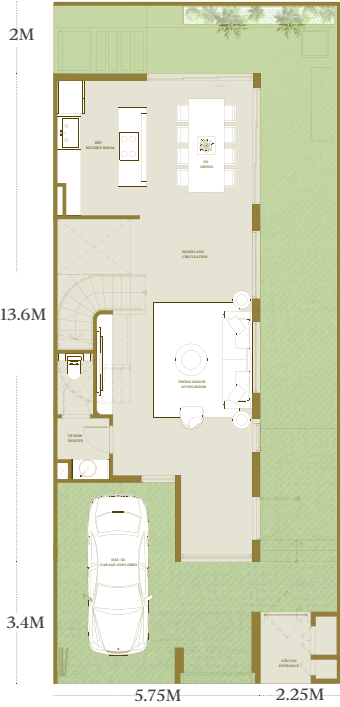
TẦNG 1 LEVEL 1
