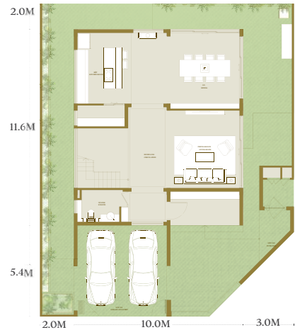
TẦNG 1 LEVEL 1
