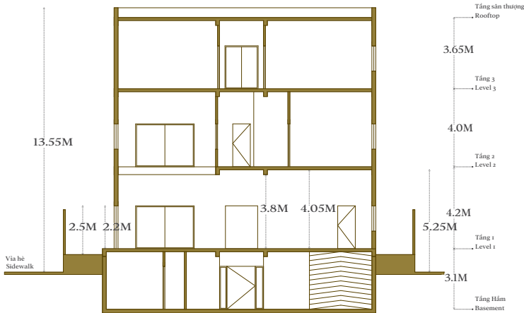
MẶT CẮT SECTION
