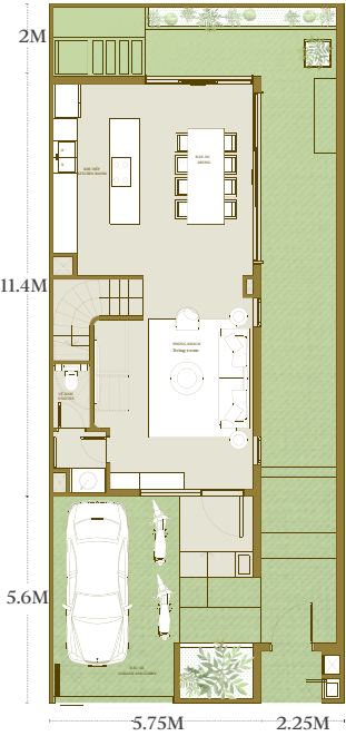
TẦNG 1 LEVEL 1
