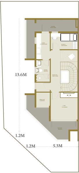
TẦNG 4 LEVEL 4
