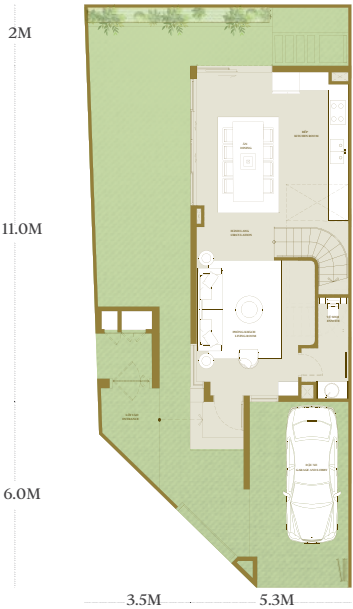
TẦNG 1 LEVEL 1
