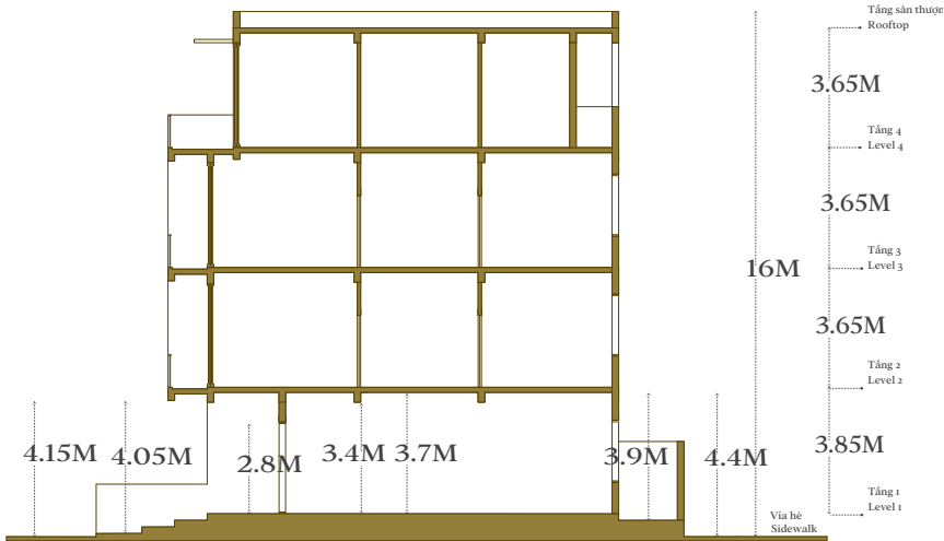
MẶT CẮT SECTION
