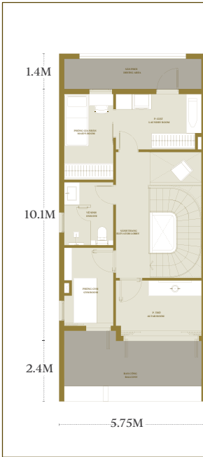
TẦNG 4 LEVEL 4
