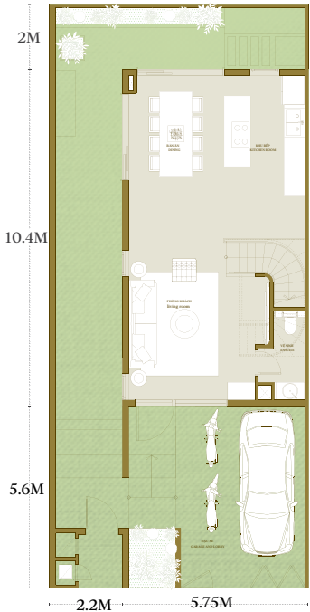
TẦNG 1 LEVEL 1
