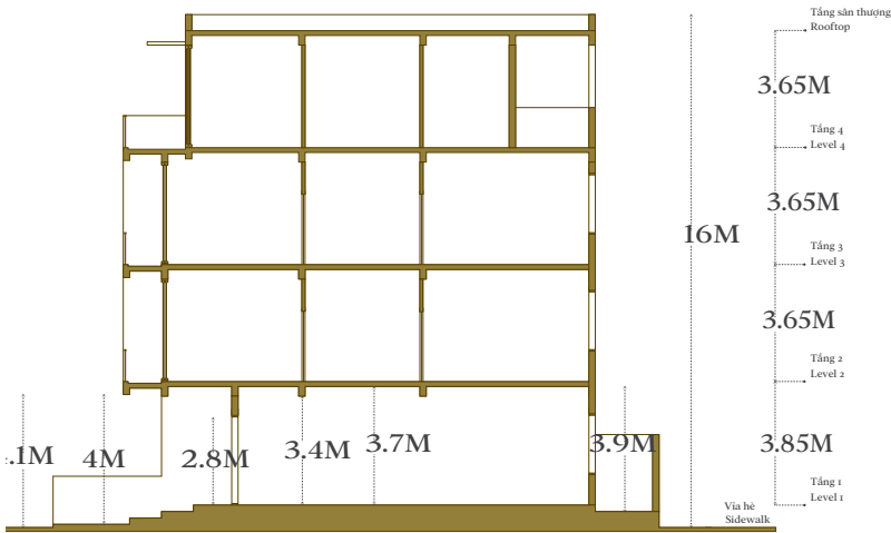
MẶT CẮT SECTION
