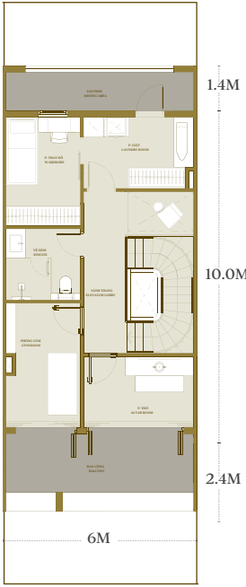
TẦNG 4 LEVEL 4
