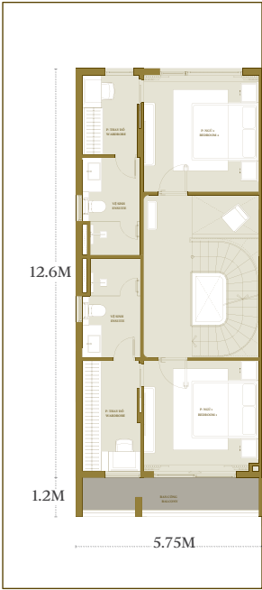
TẦNG 2 LEVEL 2
