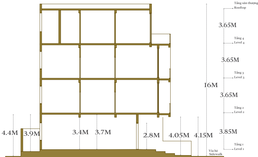
MẶT CẮT SECTION
