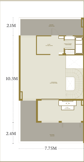
TẦNG 4 LEVEL 4
