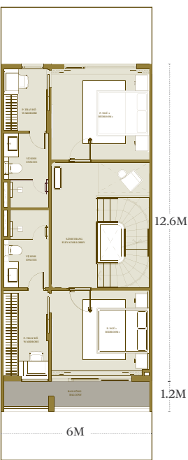
TẦNG 2 LEVEL 2
