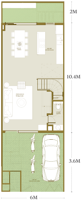
TẦNG 1 LEVEL 1
